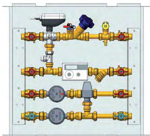
Modello IVR 483 in cassetta con miscelazione
