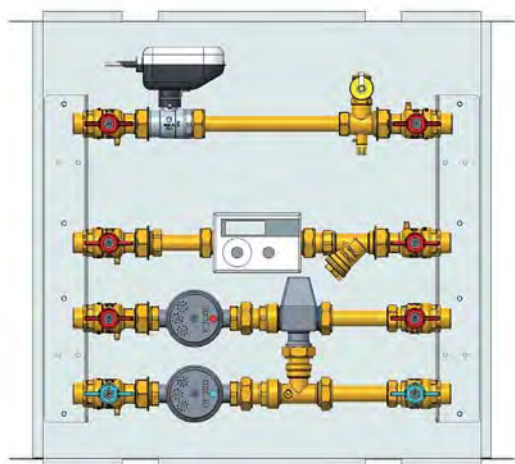
Modello IVR 472 in cassetta con miscelazione
