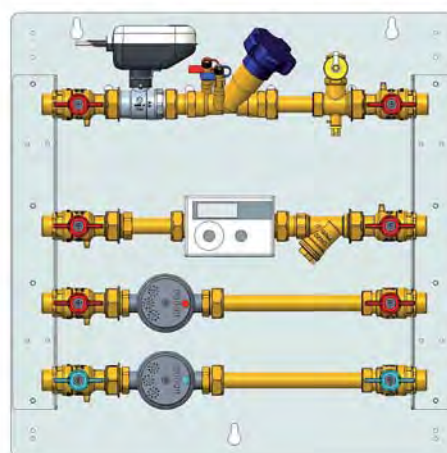
Modello IVR 482 su piastra senza miscelazione
