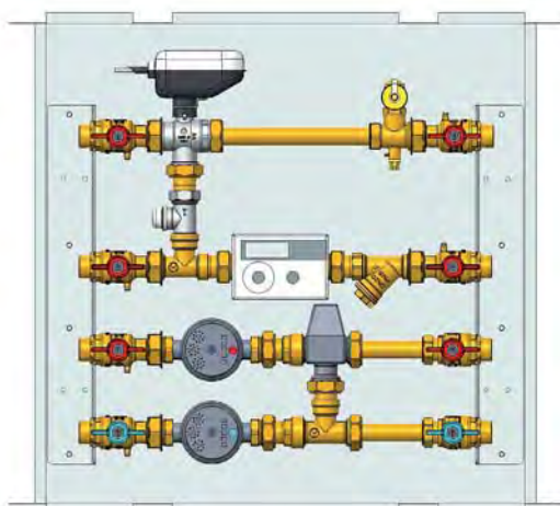
Modello IVR 473 in cassetta con miscelazione
