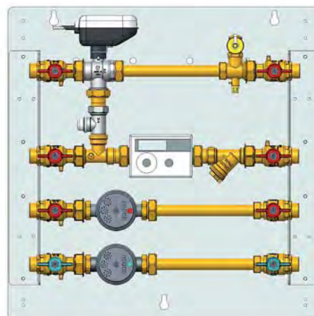
Modello IVR 473 su piastra senza miscelazione
