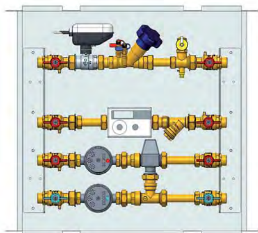
Modello IVR 482 in cassetta con miscelazione
